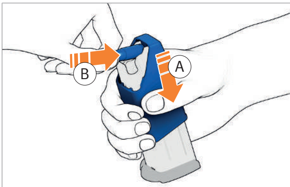
Abb. 50: Patrone unter die Magazinlippen schieben
