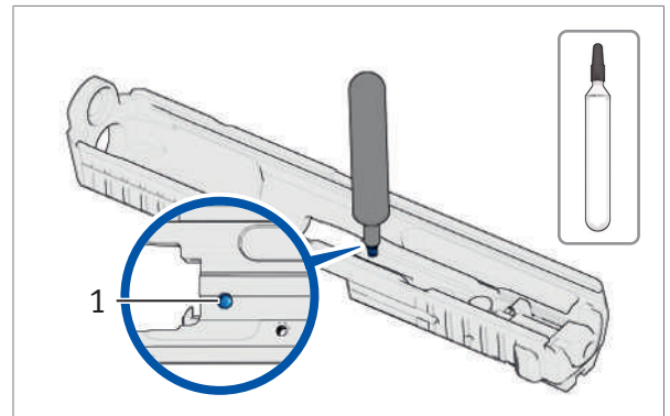
Abb. 65: Schlagbolzenbohrung mit Öl spülen
