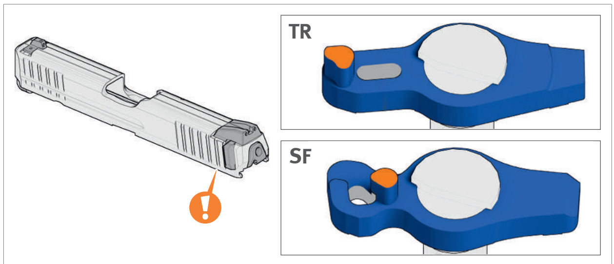
Abb. 16: Schlagbolzensicherung im Verschluss
