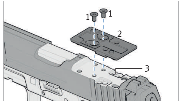
Abb. 41: Adapterplatte
