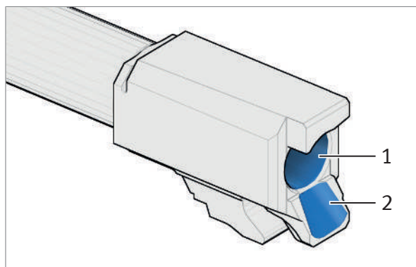
Abb. 52: Rohr, Patronenlager und Führungsfläche reinigen und entölen
