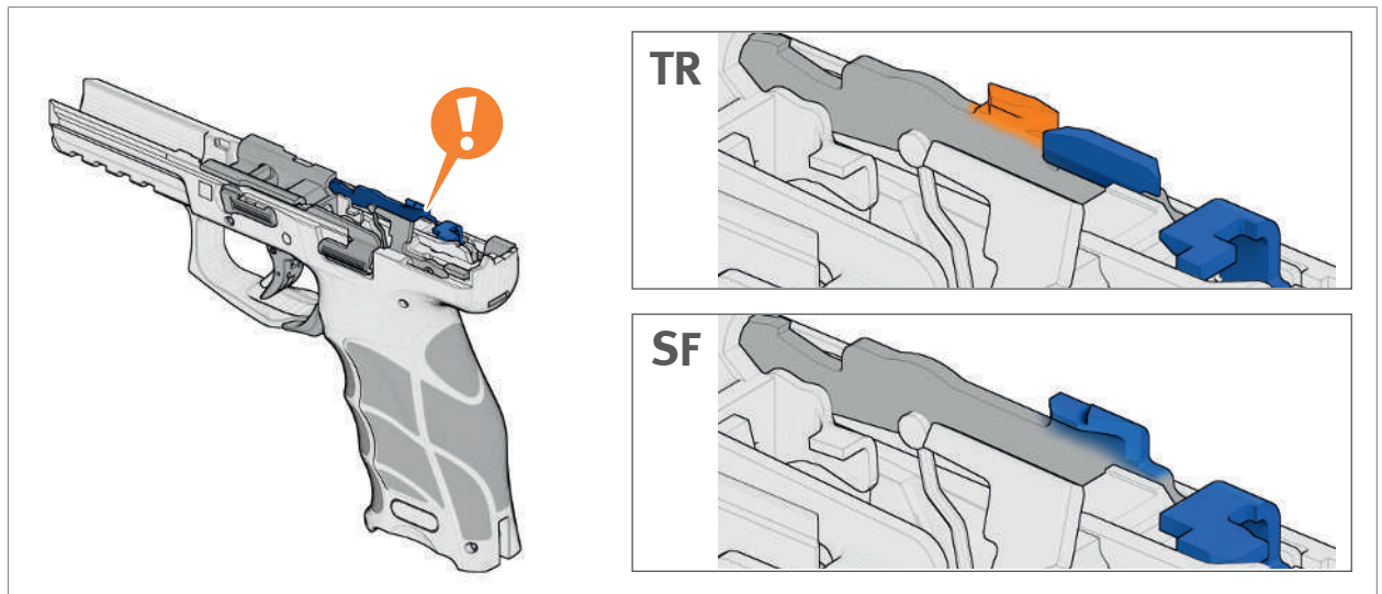
Abb. 15: Abzugsstange im Griffstück
