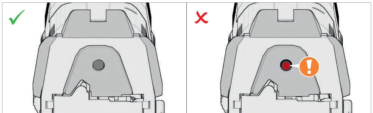
Abb. 19: Spannanzeige für Schlagbolzen
