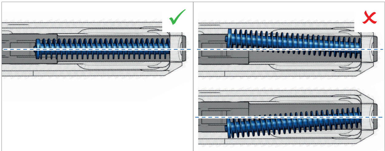
Abb. 69: Einbaulage der Schließfeder
