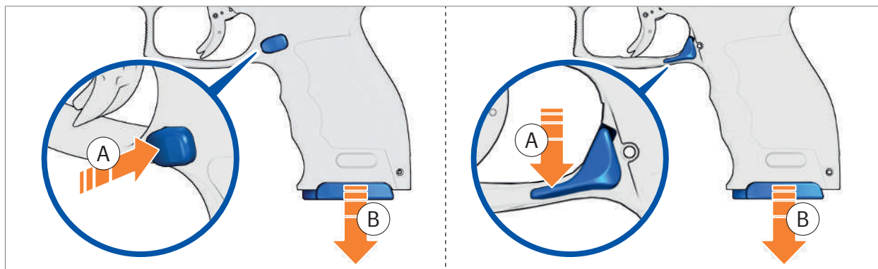
Abb. 57: Magazin entnehmen
