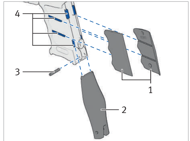
Abb. 24: Griff Rücken und Griffschalen
