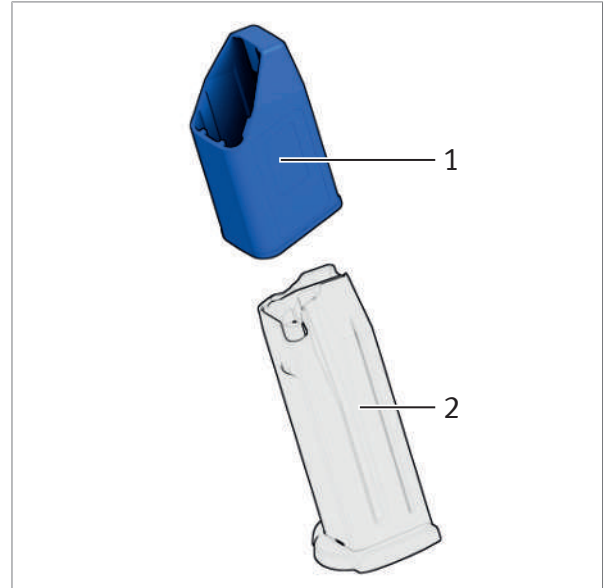
Abb. 49: Ladehilfe auf das Magazin setzen
