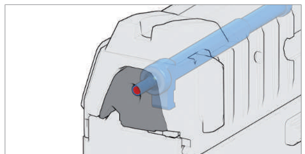
Abb. 12: Spannanzeige für Schlagbolzen
