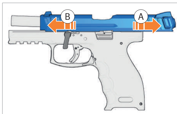
Abb. 61: Verschluss vom Griffstück schieben
