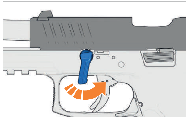
Abb. 71: Demontagehebel gegen den Uhrzeigersinn drehen
