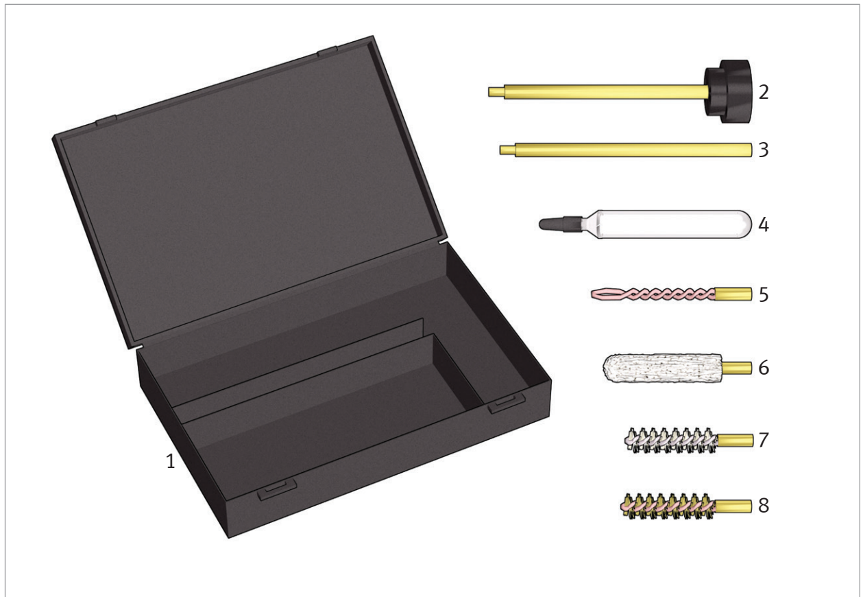
Abb. 17: Reinigungsgerät (Ident.-Nr. 988426)
