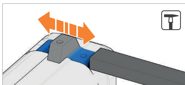
Abb. 47: Korn seitlich verschieben
