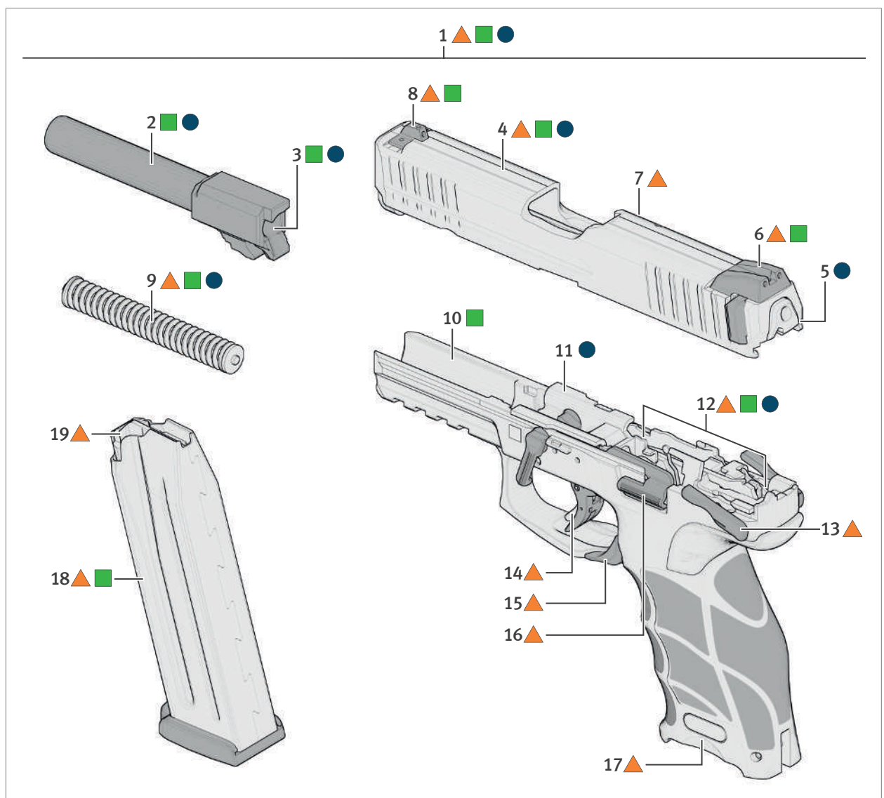
Abb. 59: Übersicht der Wartungsstellen
