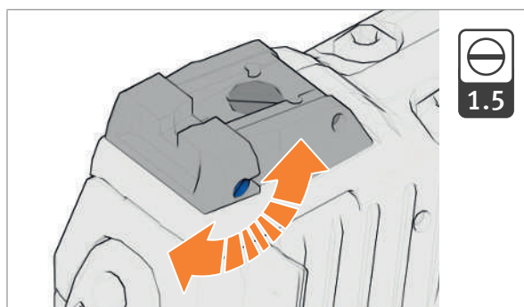
Abb. 44: Seitenjustierschraube drehen
