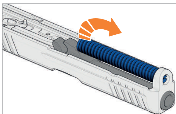
Abb. 62: Schließfeder entnehmen
