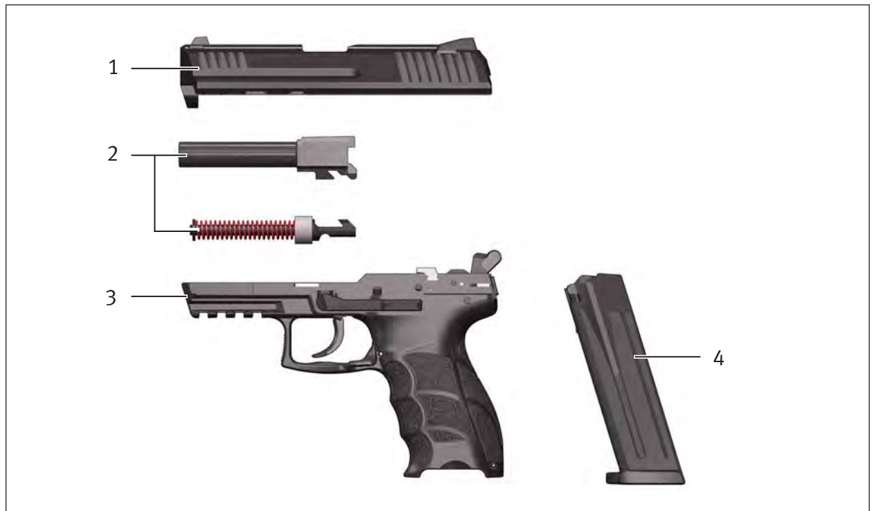
Abb. 12a: Baugruppen
