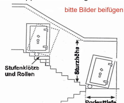
6. Treppe mit 180° angewinkelt mit Podest
